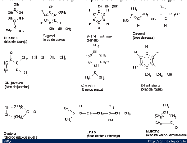
Quadro 1: apresenta as fórmulas dos principais componentes de alguns óleos essenciais.
