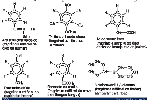
O Quadro 2 apresenta as estruturas de alguns compostos sintéticos usados em perfumaria.
