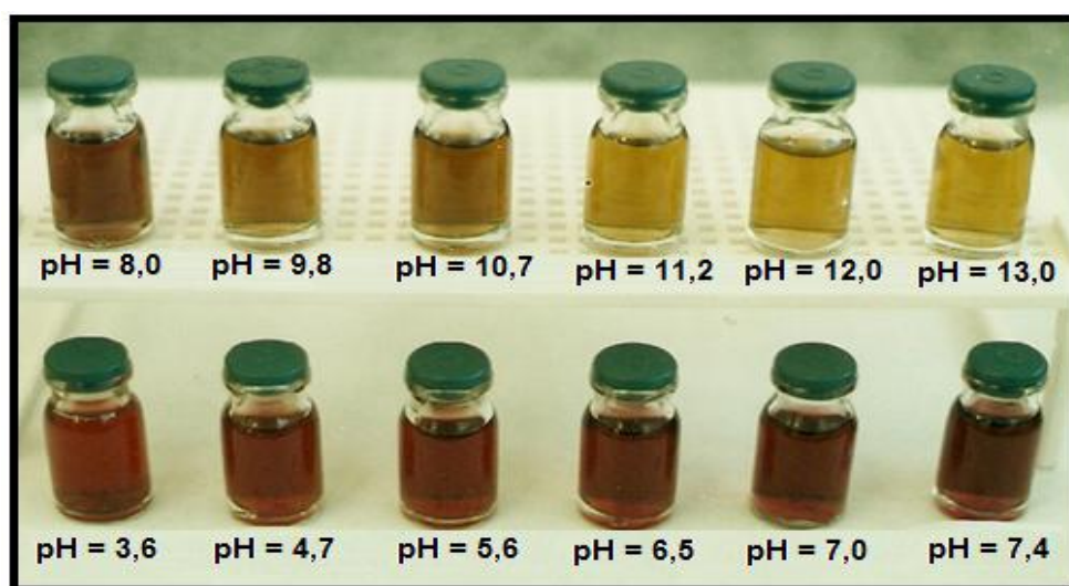
Figura 3. Escala de variação de cor do extrato da beterraba em função do pH.
