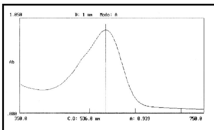
Figura 1. Espectro de UV-Visível para o extrato bruto da beterraba em meio aquoso.
