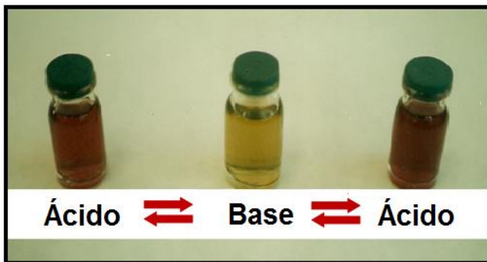
Figura 4. Mudança de caráter ácido para básico e vice-versa.
