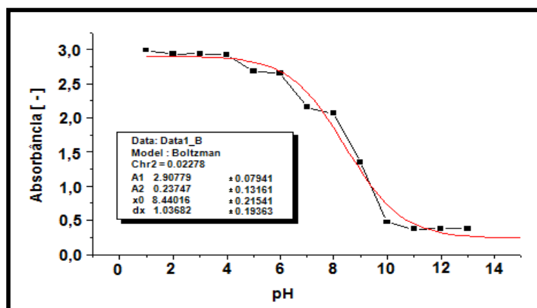
Figura 5. Curva da absorbância em função do pH para determinação do pK do indicador natural, obtida a 564 nm.
